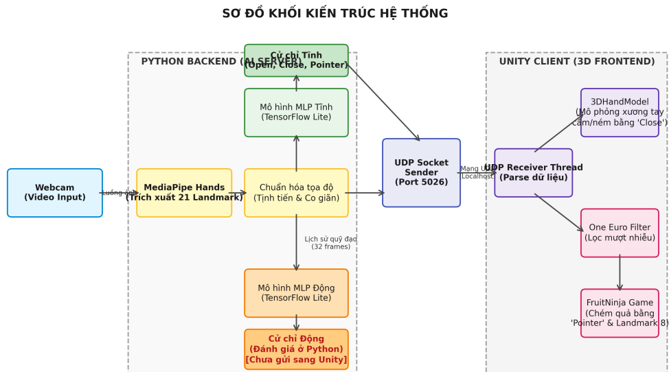
Hình 3.1: Sơ đồ khối kiến trúc hệ thống tương tác cử chỉ tay thời gian thực
