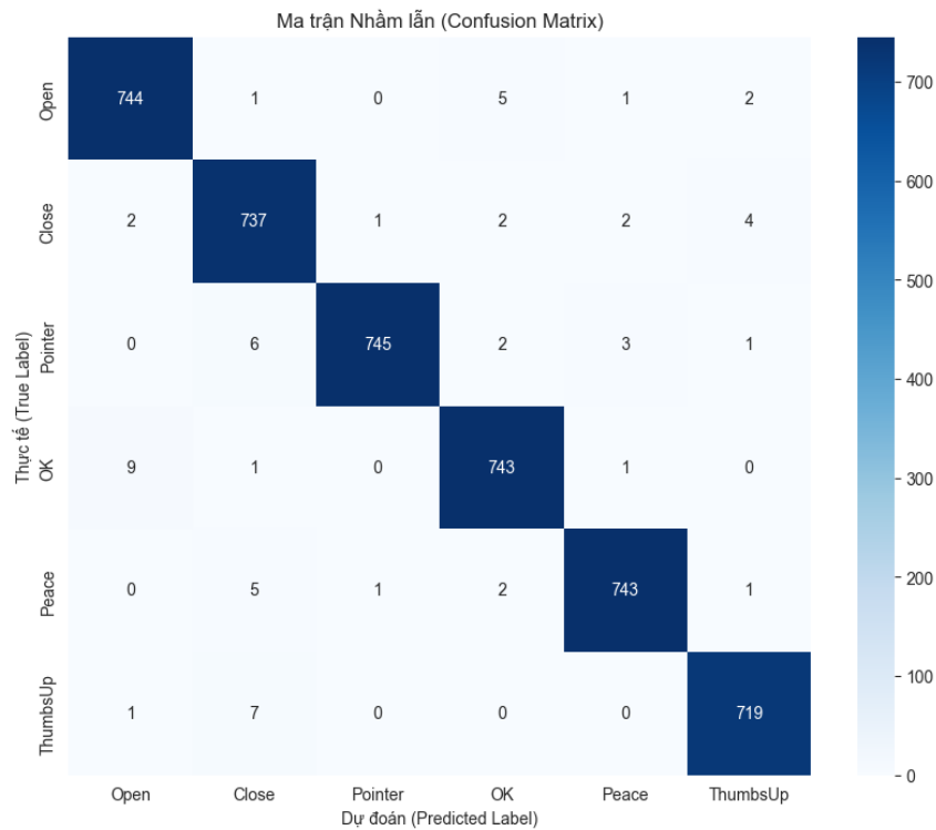
Hình 3.2: Ma trận nhầm lẫn của mô hình phân loại cử chỉ tĩnh
