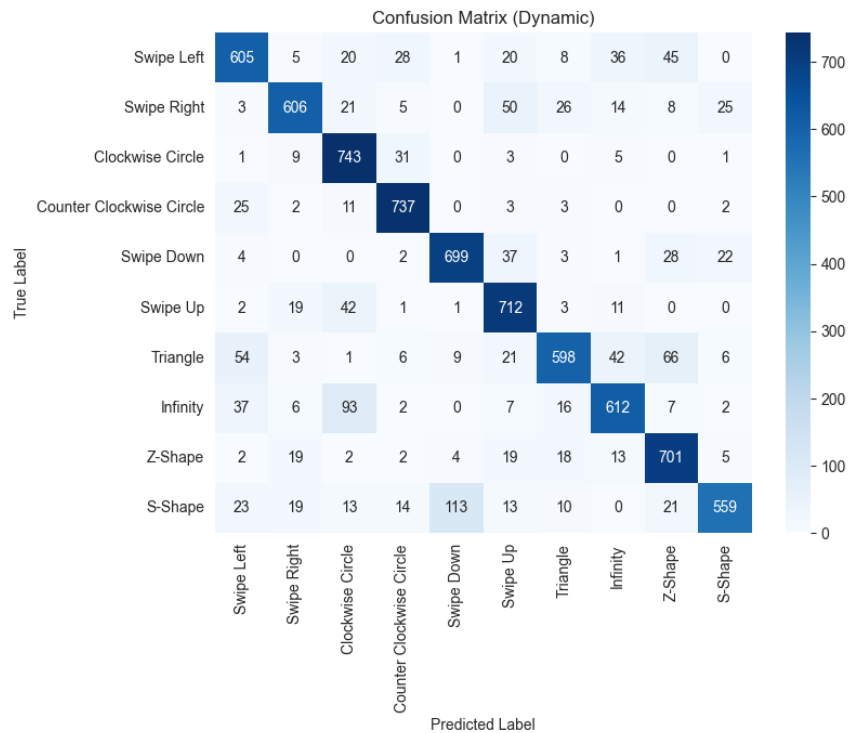
Hình 3.3: Ma trận nhầm lẫn của mô hình phân loại cử chỉ động
